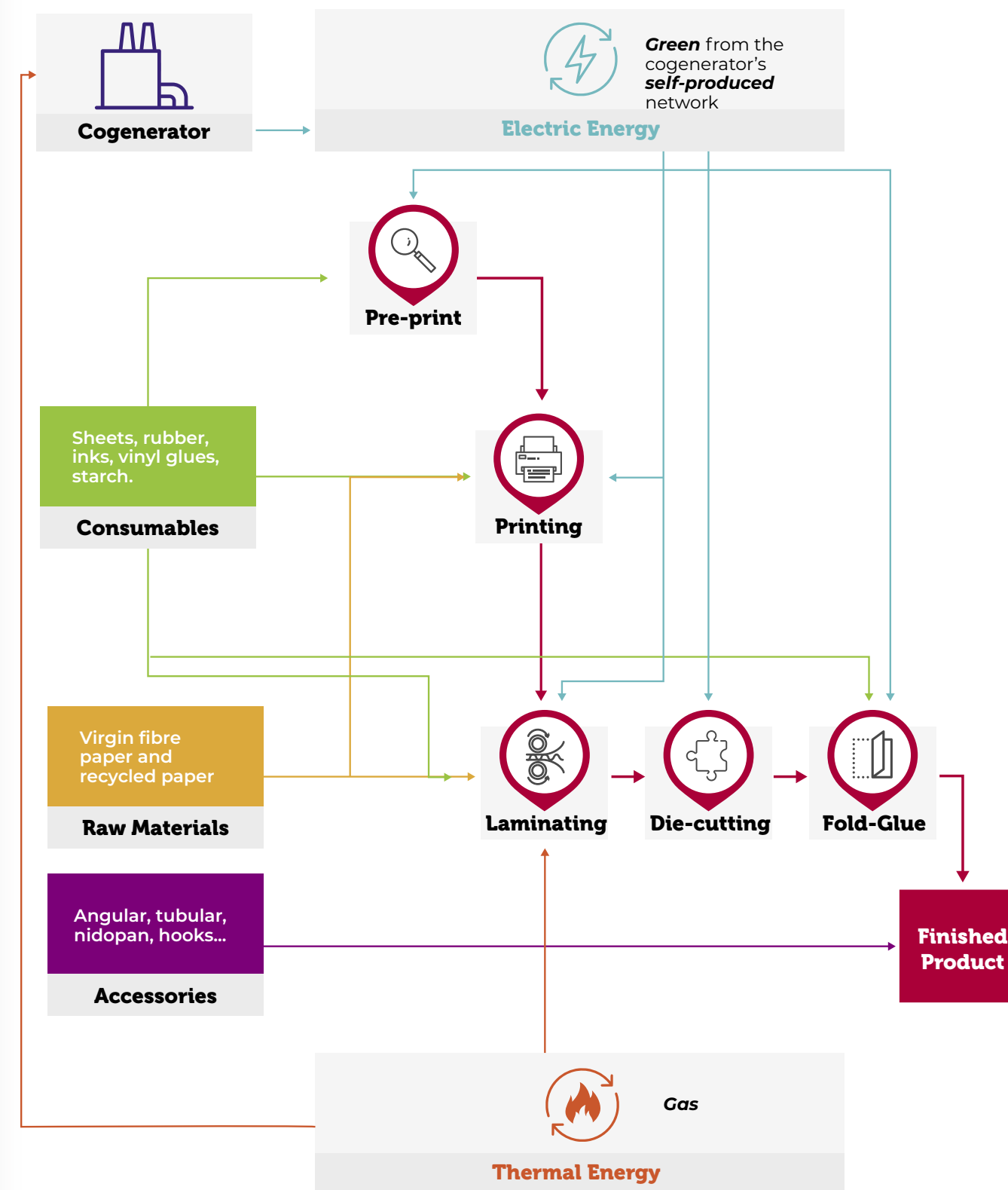
Figura 20: Schema dei processi unitari e dei flussi elementari del sistema funzionale di trasformazione Fag Artigrafiche
